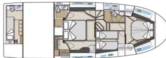
LOWER DECK WITH SKIPPER CABIN PONT INFERIEUR AVEC CABINE SKIPPER
