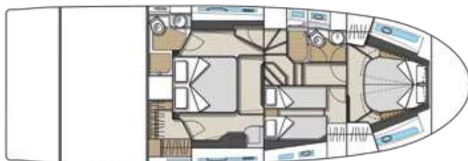
LOWER DECK - PONT INFERIEUR
